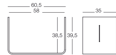
Stacking module
