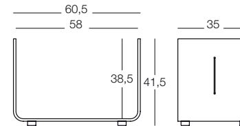
Basic module
